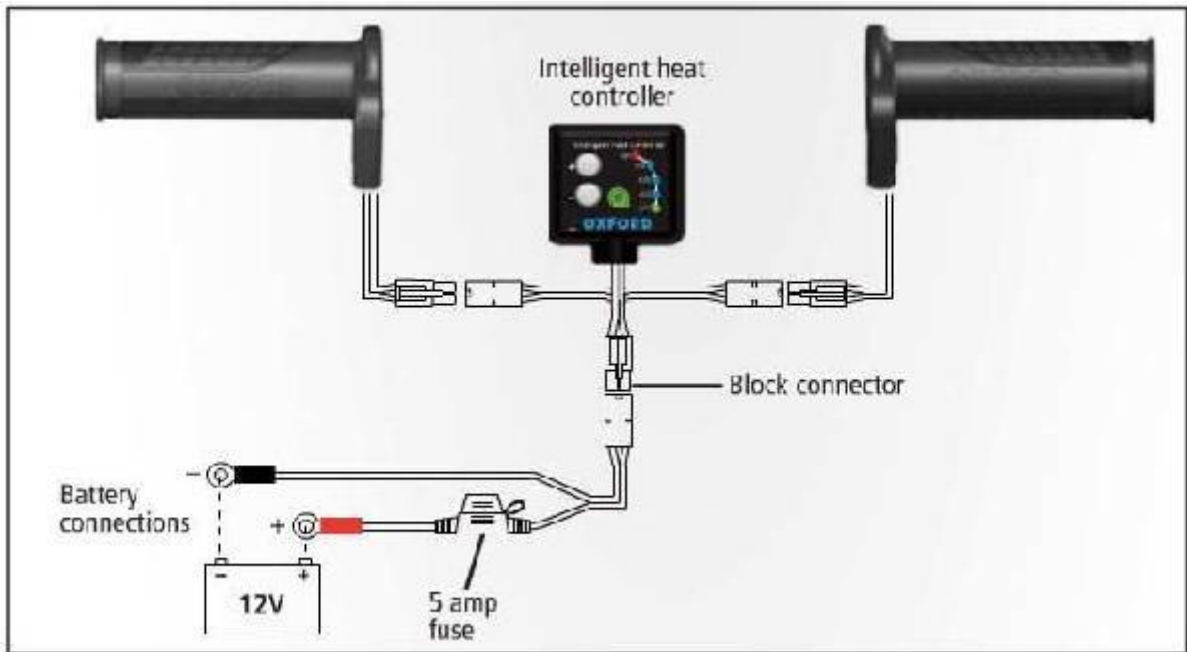
Diagram zapojení kabeláže
